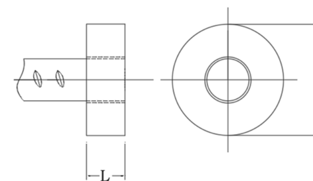
Анкерное соединение с помощью муфт DE-E
