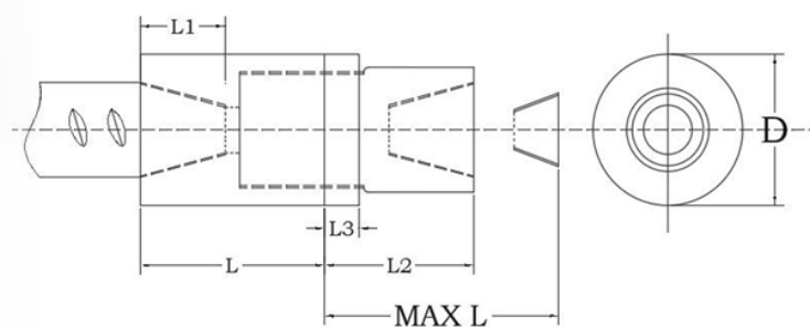
Позиционное соединение с помощью муфт DEO-P и DEO-PS
