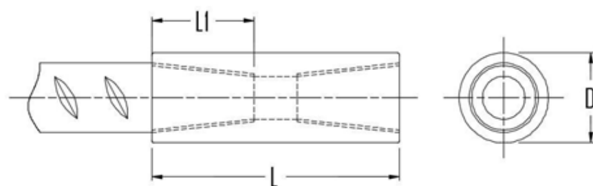
Позиционное соединение с помощью муфт DEO-A
