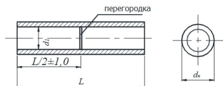
Стандартное соединение с помощью муфт DP
