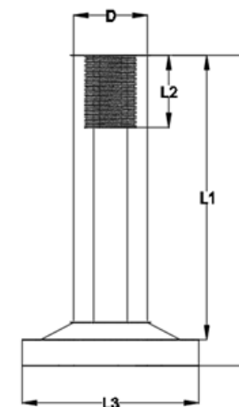
ГЕОМЕТРИЧЕСКИЕ ПАРАМЕТРЫ СОЕДИНЕНИЙ (DE-N)
