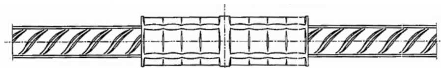
Растянутое соединение, опрессованное с промежутками
