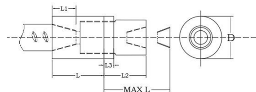
Переходно-Позиционное соединение с помощью муфт DEO-TP
